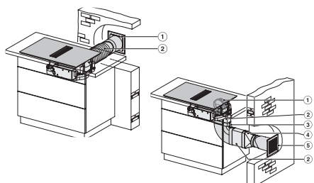
DFKS-AR Fladkanalsæt til udluftning til det fri.
